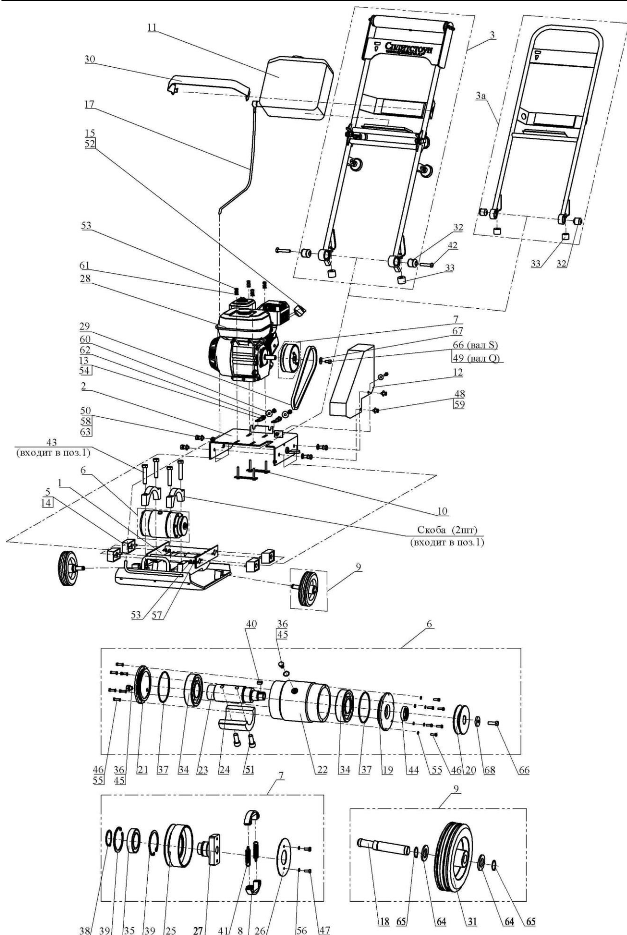
Рисунок 8 – Компоновка виброплиты
